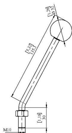
Handle M10
